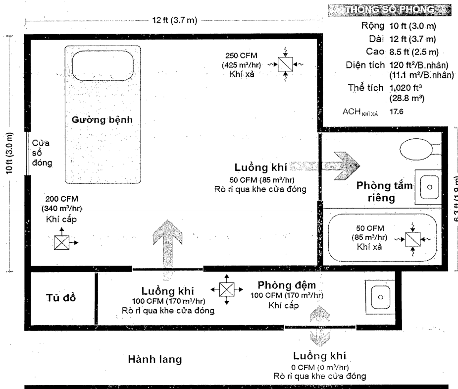
Hình 9.2: Mẫu một phòng cách ly hô hấp có phòng đệm 27
